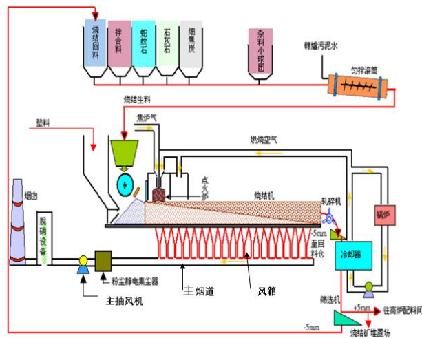
图 1 烧结工艺流程图
